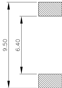
PCB Layout(Pattern side)
